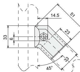
Conector Externo de 45°
