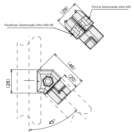
Conector interno de 45°
