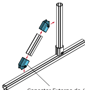
Conector Externo de 45°
