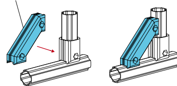
Conector de Ponto
